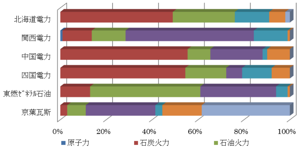
電気小売事業者の電源構成 (2015年度実績)
